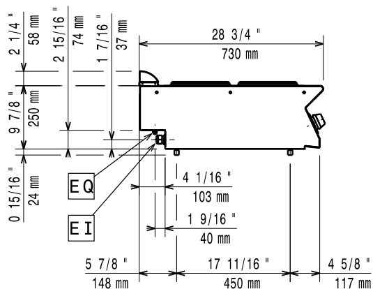
Oldalnézet
